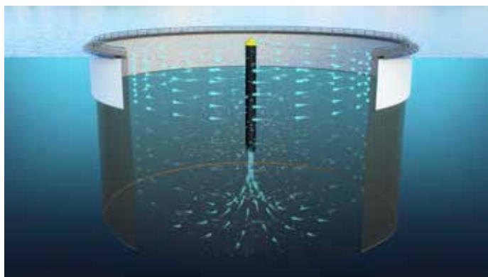
Framo AquaStream er en type systemløsning for merder med luseskjørt. Med en Framo SR2000 strømsetter pumper vi store mengder friskt vann opp i luseskjørtet, og fordeler vannet slik at vannutskiftingen skjer på en mest mulig effektiv måte.
